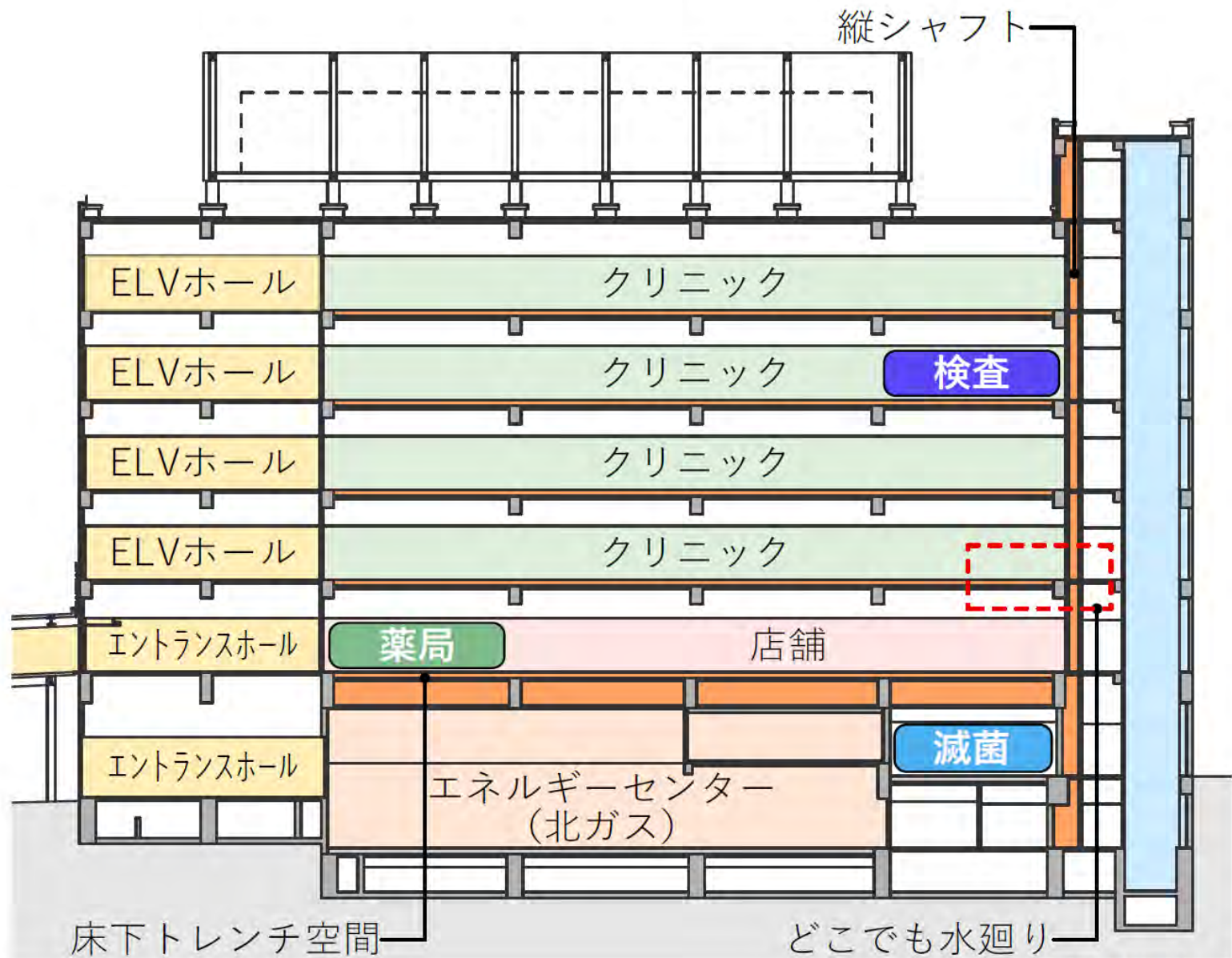
断面構成図
